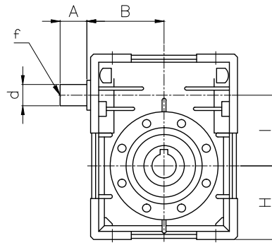
BVS 063-075-090
