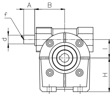
BVS 030-040-050
